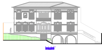
Elevation 01
