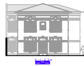
Elevation 02
